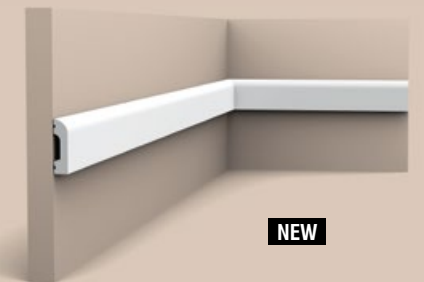
DX182-2300 | D182F CASCADE 230 x 5 x 1,3 cm (DX182-2300) Duropolymer ® 200 x 5 x 1,3 cm (DX182F)
